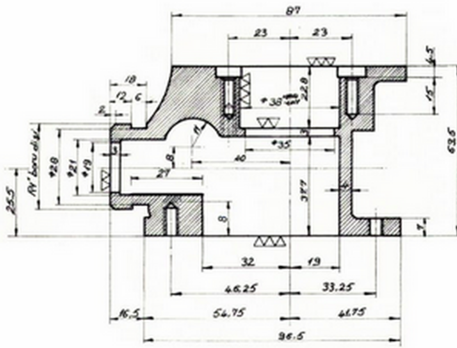
A-A KESİTİ
